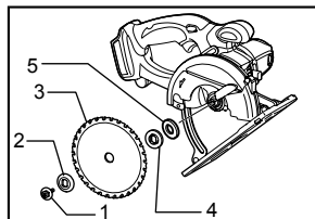
1. Perno hexagonal 2. Brida exterior 3. Disco de sierra 4. Brida interior 5. Arandela cóncava
