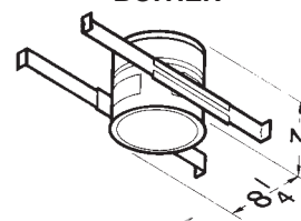
MODÈLE 505 BOÎTIER
