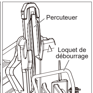
LOQUET DE DÉBOURRAGE OUVERT
