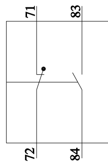
Rechts / right
