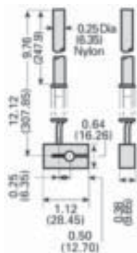
Nylon Spring Rod Actuator 3SX03-KL556
